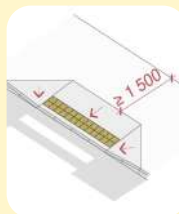
Приклад влаштування бордюрного пандусу (розміри вказані у мм)
